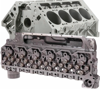
كتلة الأسطوانات ورأسها Cylinder Block & Head
